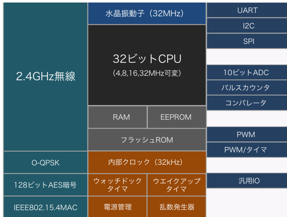
図 4 BLUE PAL/RED PAL のブロック図
