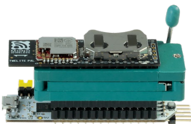
図 3 TWELITE R との接続例 2
