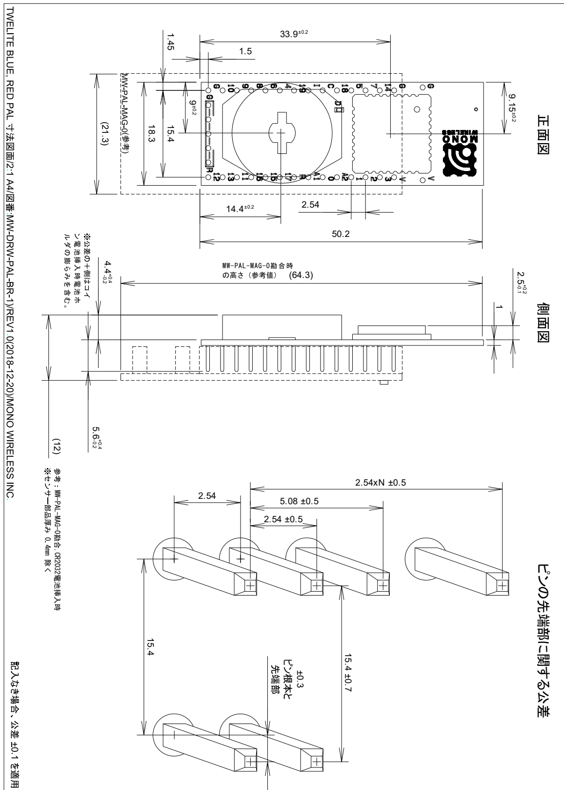
図 5 外形寸法図
