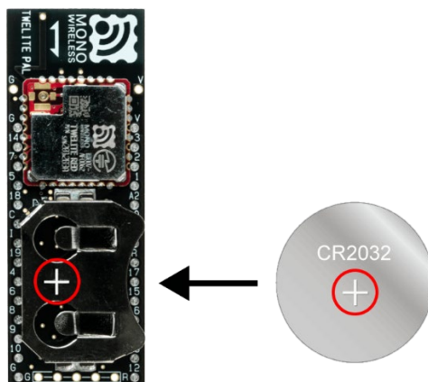
図 1 コイン電池の挿入方法
