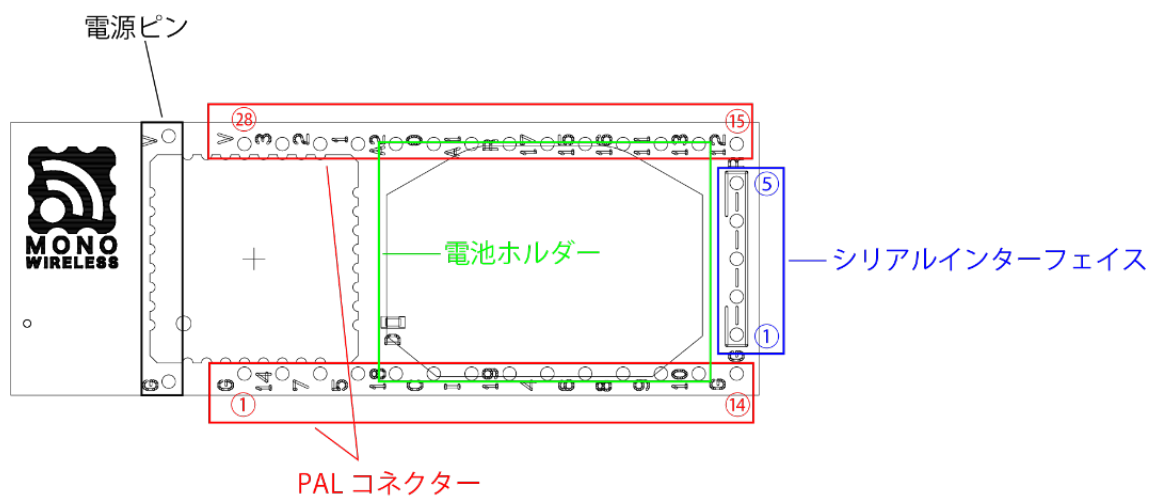
図 6 ピン配置図
